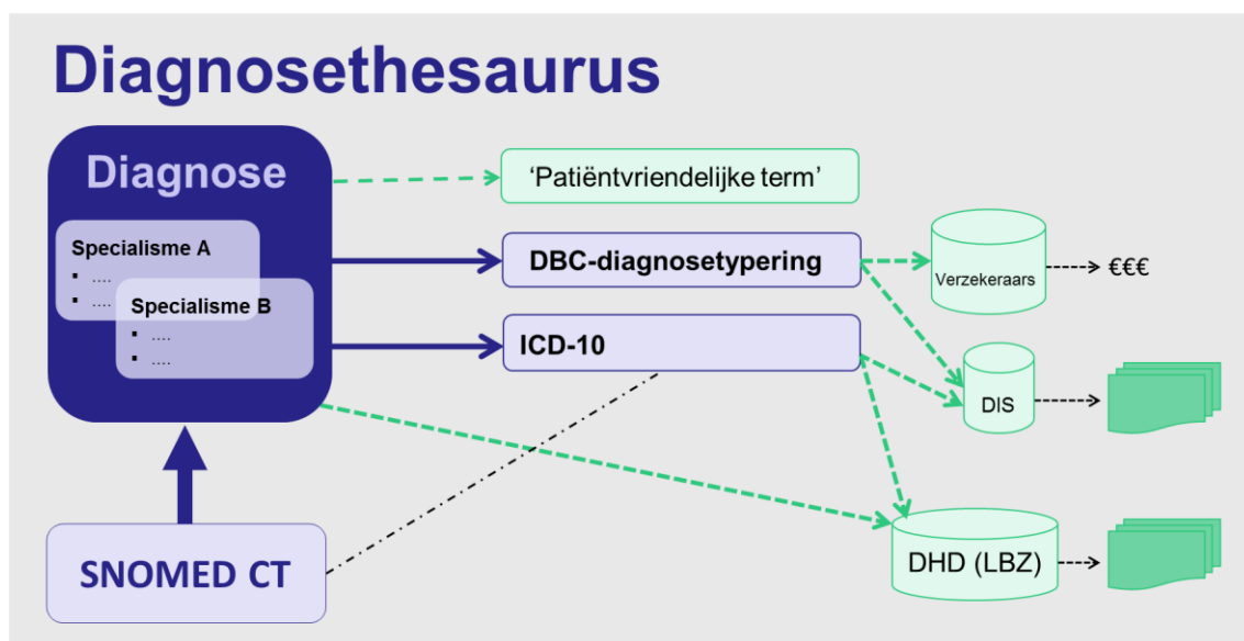
Figuur 1 Schematische weergave van de Diagnosethesaurus met directe afleidingen in scope van de Diagnosethesaurus (paarsblauwe lijnen).
